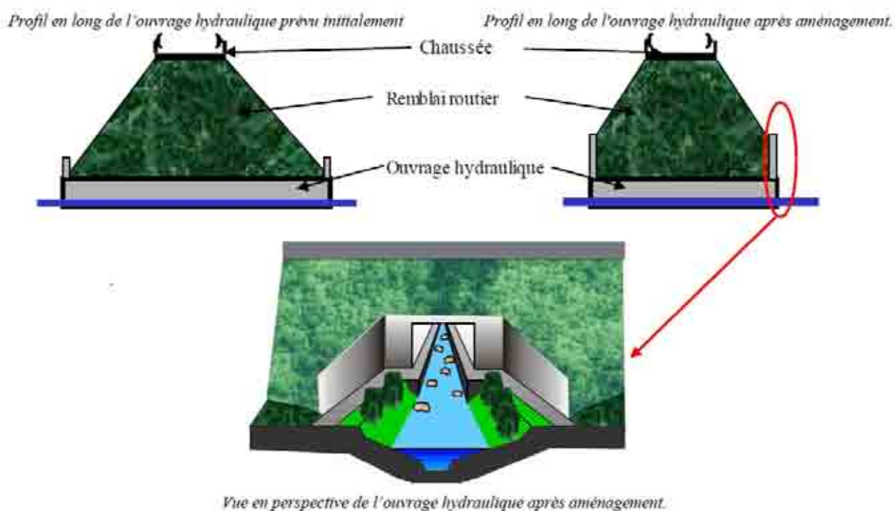
Figure 6 : Principe de r duction des longueurs d'ouvrage et d'am nagement de leurs d bouch s.
