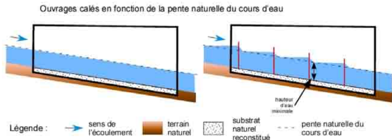
Figure 3 : profils en long de cours d'eau et ouvrages hydrauliques fermés (OH) : exemple d'ouvrages respectant la pente naturelle du cours d'eau, à équiper dès lors que les vitesses deviennent supérieures à la capacité de nage des poissons.
