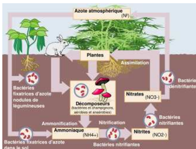
Figure 14 : le cycle biogéochimique de l'azote – J. Dréo 2006
