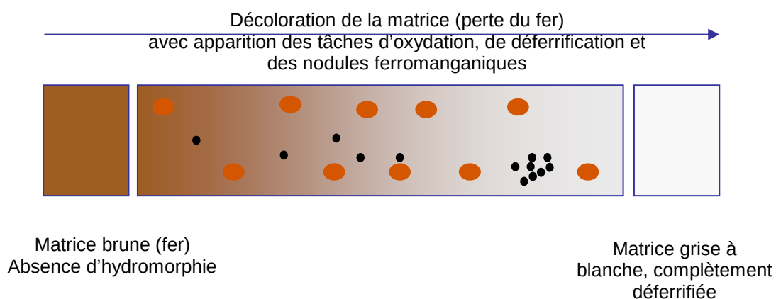
Figure 7 : progression de l'hydromorphie
