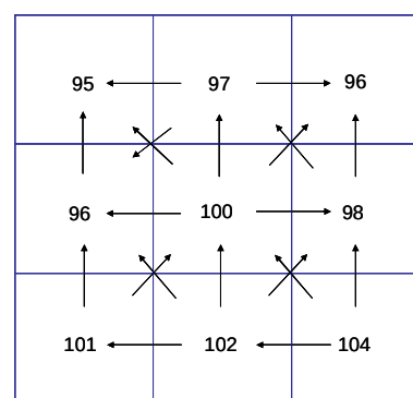
Figure 5 : exemple de modèle de drainage multi-directionnel (d'après Aurousseau et Squivadent, 1995)
