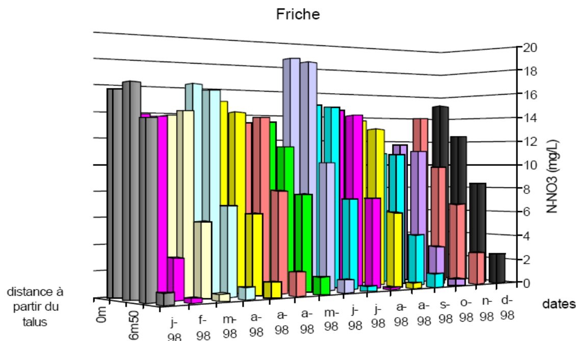
Figure 2: Décroissance des concentrations en nitrate dans l'eau de subsurface à l'interface versant – zone humides (Clément, 2000).
