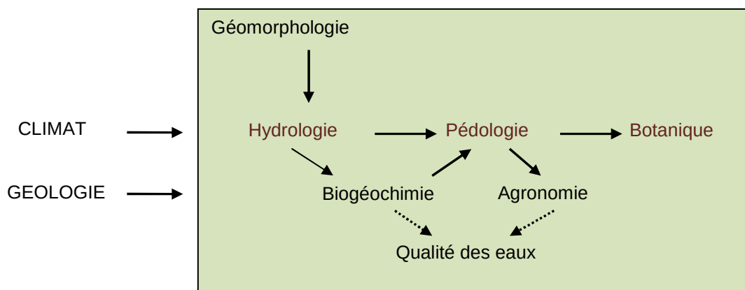
Figure 4 : schéma conceptuel des relations entre les critères de caractérisation des zones humides (Mérot et al. 2000)
