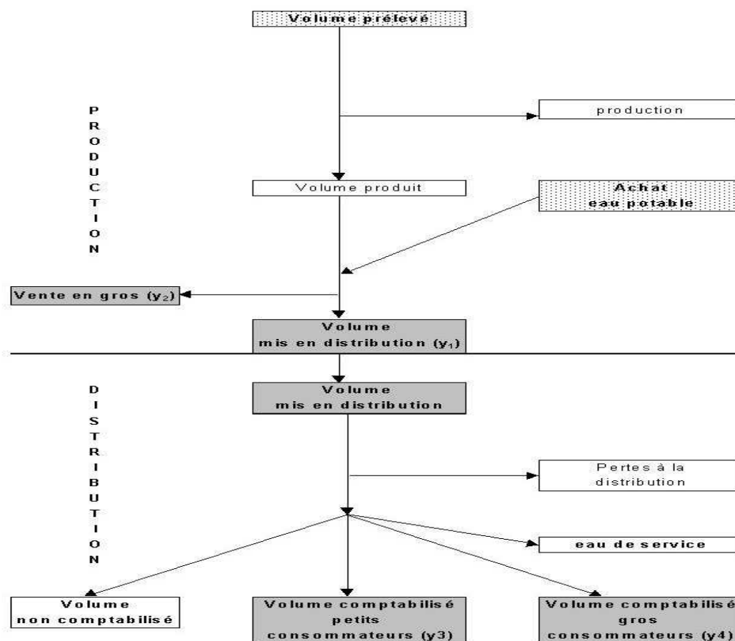
FIG. B.2 – Les volumes d'eau en circulation
