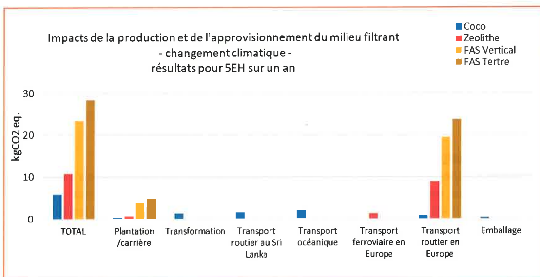
FIGURE 3 – IMPACTS ANNUELS DE LA PRODUCTION DES MATERIAUX DU MILIEU FILTRANT - INDICATEUR CHANGEMENT CLIMATIQUE
