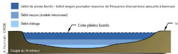
Schéma de profil – débit et cote
