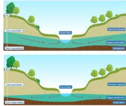
Des échanges entre les nappes souterraines et les cours d'eau OFB (Matthieu Nivesse, d'après OIEau), 2018
