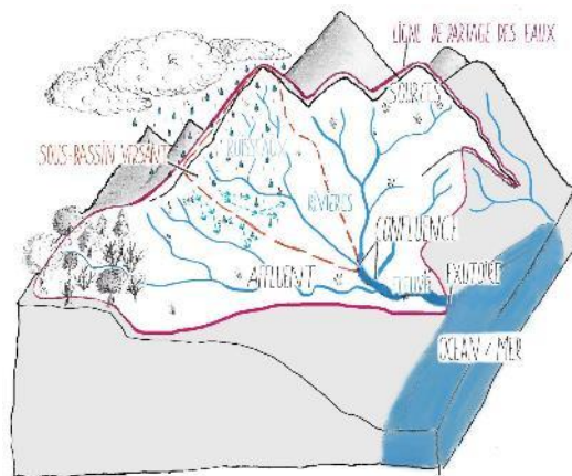
Le bassin versant Association du Réseau des Sites Rivières Sauvages, 2020
