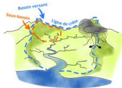
Bassin versant et sous-bassin versant Office International de l'Eau - OIEau, 2019
