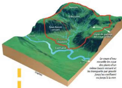
Le bassin versant OFB, 2012
