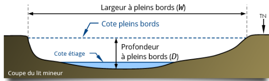
Profil de cours d'eau Xavier FOURNIALS – CATER-COM, 2018
