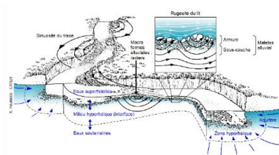
Les écoulements hyporhéiques Xavier FOURNIALS – CATER-COM, 2018
