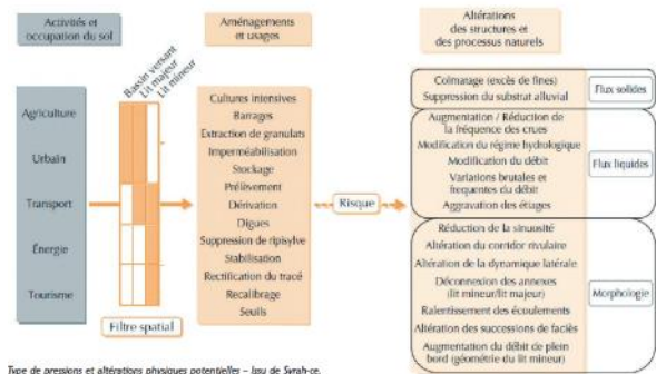
Type de pressions et altérations physiques potentielles – issu de Syrah-co OFB, 2018
