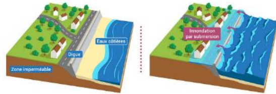
L'inondation par submersion OFB (Matthieu Nivesse, d'après OIEau), 2018
