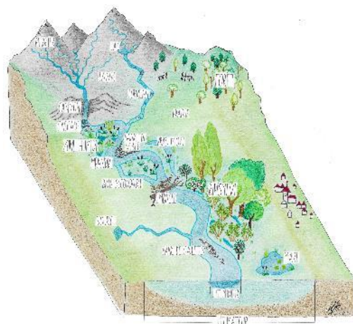
La mosaïque d'habitats d'une rivière sauvage Association du Réseau des Sites Rivières Sauvages, 2020
