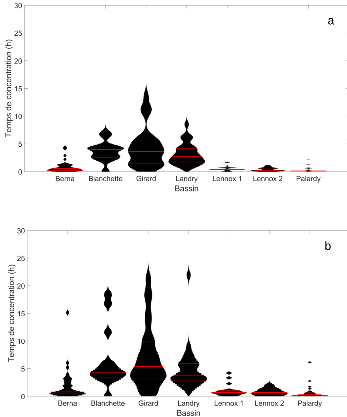
Figure 4.5 - Distribution ( violin plots ) des valeurs des temps de concentration selon la méthode d'estimation : a) PNDP et b) T_P . La ligne rouge centrale correspond à la médiane et les deux traits fins rouges correspondent aux 25 e et 75 e percentiles de la distribution empirique.
