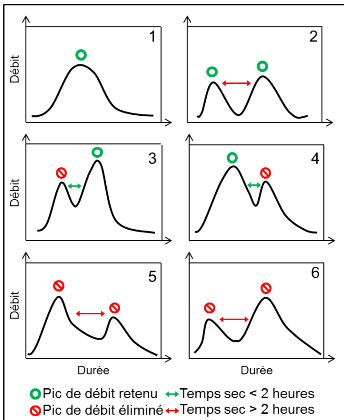
Figure 3.2 - Exemples d'hydrogrammes observés (voir le texte pour une discussion de ces différents cas).
