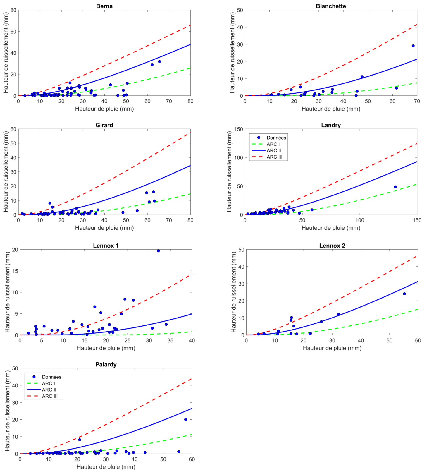
Figure 5.4 – Hauteur de ruissellement (mm) en fonction de la hauteur de pluie (mm) aux sites sous étude. Les courbes correspondent à la Méthode SCS modifiée (ARC I, II et III) et les points aux valeurs mesurées aux différents sites.
