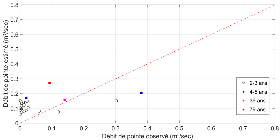
Figure 6.4 – Comparaison des débits de pointe observés et des débits de pointe estimés à partir de la méthode rationnelle en considérant le temps de concentration obtenu avec l'équation de Sheridan modifiée. La période de retour de chacun des événements de pluie est également indiquée. La ligne pointillée rouge représente la droite de pente 1.
