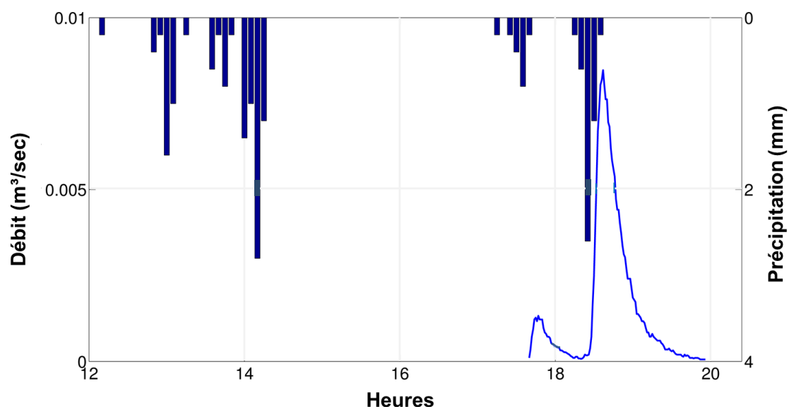
Figure 3.1 – Influence de la période de temps sec considérée à partir de l'hydrogramme et du hyétochrome de l'événement pluie/débit du 5 mai 2010 au site Berna.
