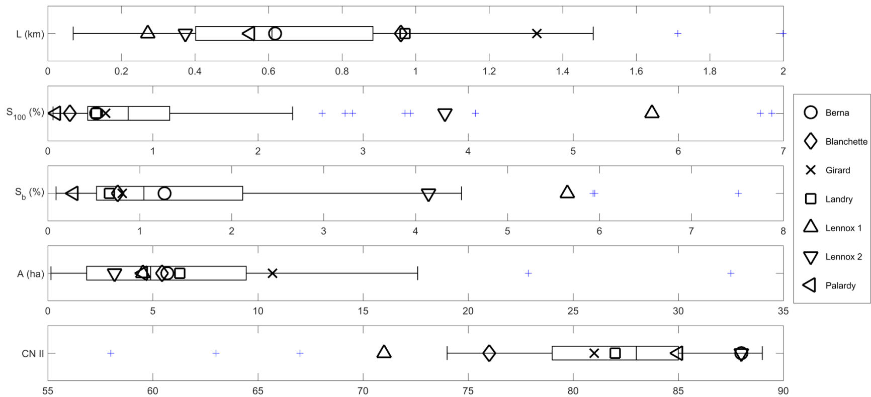
Figure 2.3 – Distribution des caractéristiques, longueur du parcours de l'eau (L, km), pente du cours d'eau ( S_{100} , %), pente du bassin-versant ( S_b , %), superficie du bassin-versant (A, ha) et numéro de courbe (CN, adimensionnel) des 50 bassins-versants caractérisés par Mikael Guillou et des bassins-versants à l'étude.
