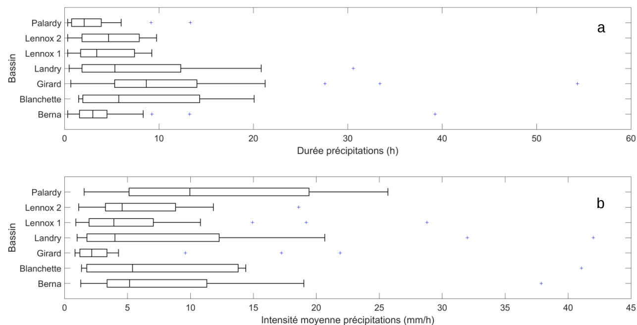
Figure 4.3 - Box plots des : a) durées, et b) des intensités moyennes des épisodes de pluie associés à des hydrogrammes simples utilisés pour l'estimation des temps de concentration sur chacun des bassins à l'étude (150 événements au total).
