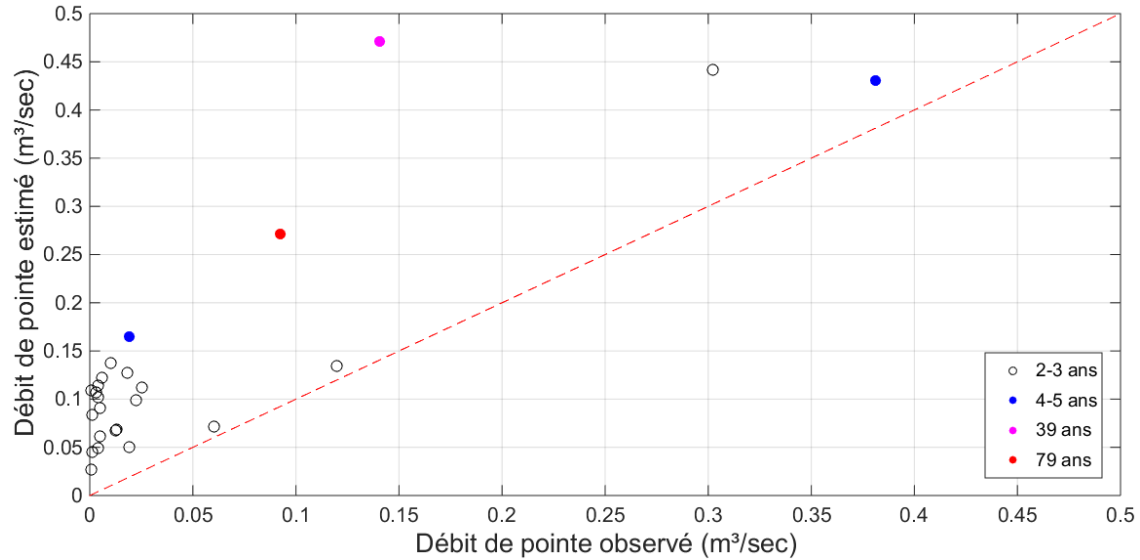
Figure 6.5 – Comparaison des débits de pointe observés et des débits de pointe estimés à partir de la MHT ajustée, considérant le temps de concentration obtenu avec l'équation de Sheridan modifiée selon la période de retour de chacun des événements pluie/débit (la ligne en rouge représente la droite de pente 1).
