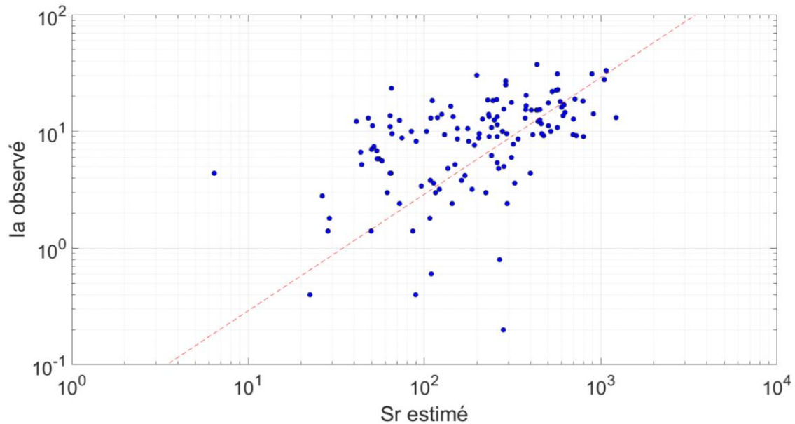
Figure 5.6 - Valeurs de S_r pour chacun des événements aux différents sites avec les valeurs correspondantes de I_a mesurées selon la procédure décrite à la Figure 5.2. La pente de la régression correspond à \lambda=0.03
