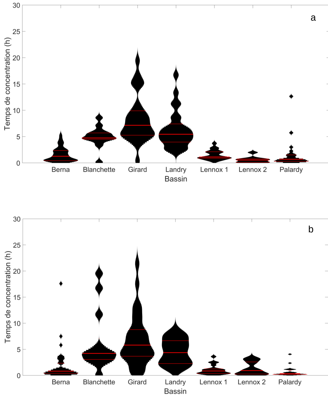
Figure 4.4 - Distribution ( violin plots ) des valeurs des temps de concentration selon la méthode d'estimation : a) CM et b) T_L . La ligne rouge centrale correspond à la médiane et les deux traits fins rouges correspondent aux 25 e et 75 e percentiles de la distribution empirique.
