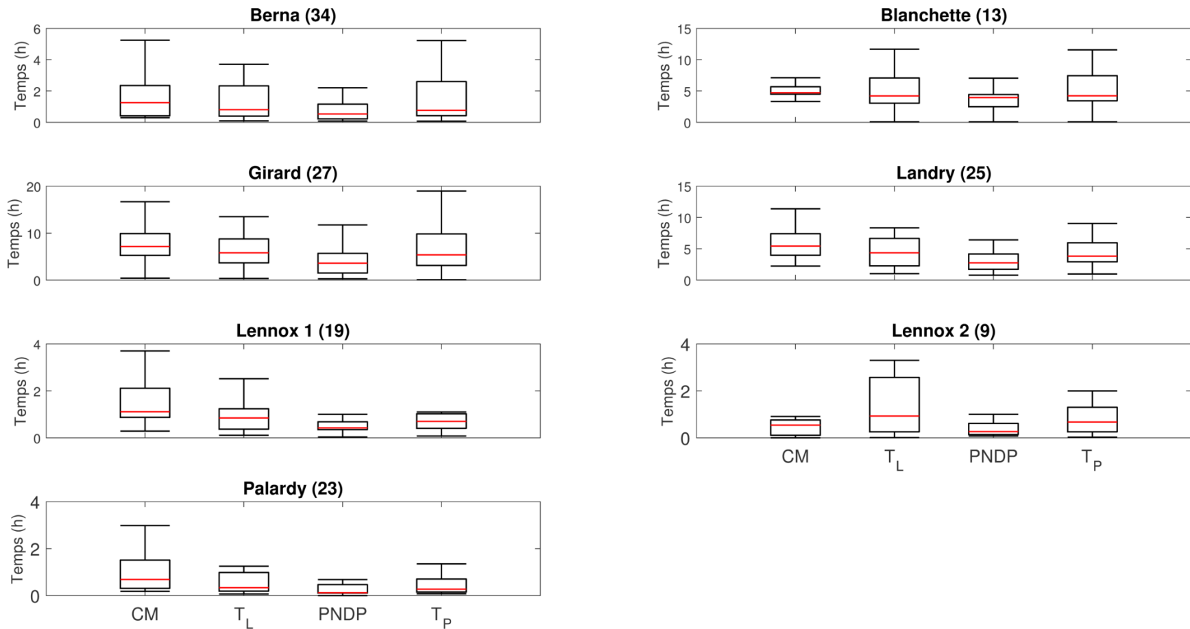
Figure 4.6 - Box plots des temps de concentration pour chacun des sites selon les quatre méthodes d'estimation retenues (ligne rouge : médiane; le nombre d'événements pluie/débit considérées est indiqué entre parenthèses). Certains temps de concentration se situant à l'extérieur des moustaches des box plots ont été volontairement retirés afin de faciliter l'interprétation des graphiques.
