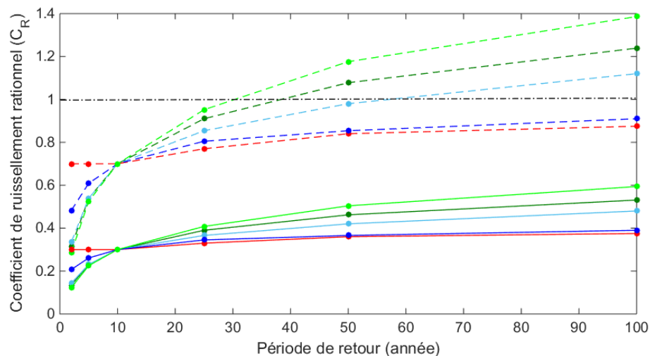
Figure 6.2 - Coefficients de ruissellement rationnels ajustés en fonction de la période de retour selon les facteurs de correction provenant de différentes études (lignes pleines : C_R = 0,30 ; lignes pointillées : C_R = 0,70 ; rouge : Gupta (1989) et Viessman et Lewis (2003); bleu foncé : Jens (1979, 65 % imperméable); bleu pâle : Jens (1979, 0 % imperméable); Vert foncé : Young et al. (2009); vert pâle : Dhakal et al. (2013b).
