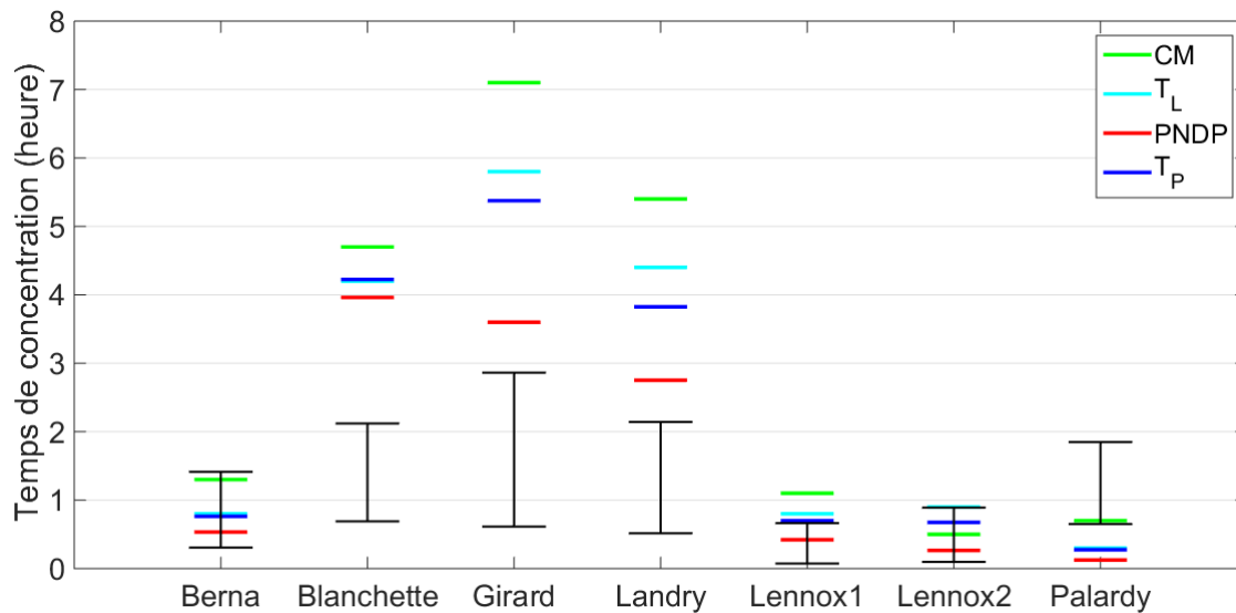
Figure 4.8 - Valeurs minimales et maximales (traits horizontaux noirs) des temps de concentrations (en heures) calculées à partir des différentes équations empiriques proposées dans la littérature et temps de concentration médians estimés à partir des quatre méthodes d'estimation des temps de concentration (CM, T L , PNDP et T P ) en chaque site.
