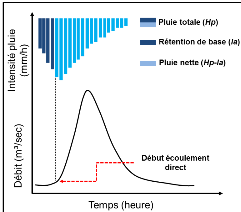
Figure 5.1 – Estimation de la rétention de base ( I_a ) à partir d'un hyétogramme et d'un hydrogramme (Source : Samuel Bolduc).
