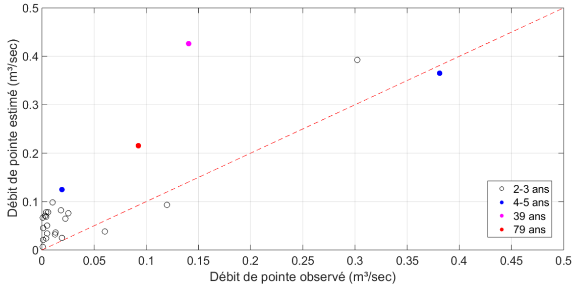
Figure 6.7 – Comparaison des débits de pointe observés et des débits de pointe estimés à partir de la MHT originelle, considérant le temps de concentration obtenu avec l'équation de Sheridan modifiée, selon la période de retour de chacun des événements pluie/débit (la ligne en rouge représente la droite de pente 1).
