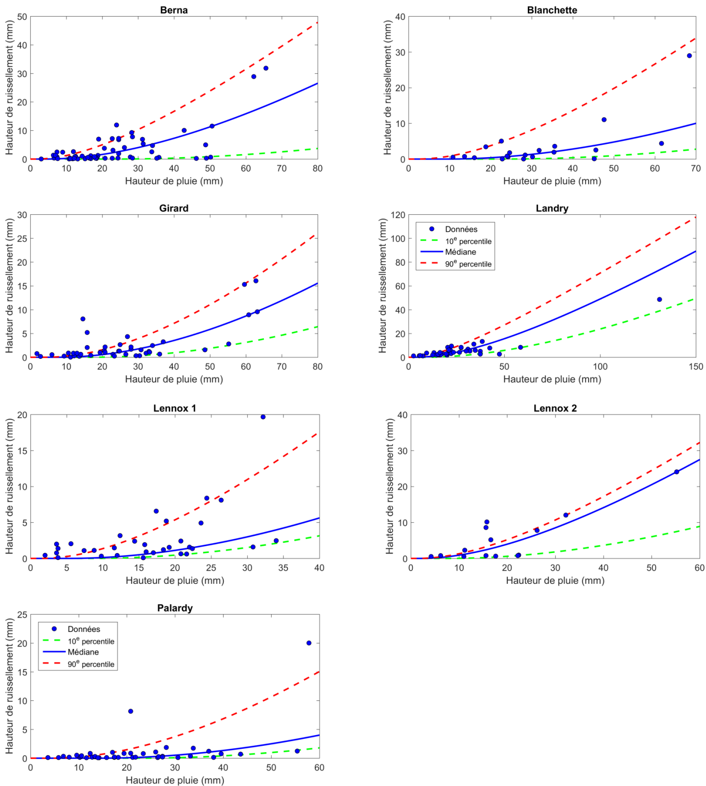
Figure 5.7 - Hauteur de ruissellement (mm) en fonction de la hauteur de pluie (mm) aux sites sous étude. Les courbes correspondent à la Méthode SCS ajustée (ARC I, II et III) et les points aux valeurs mesurées aux différents sites.
