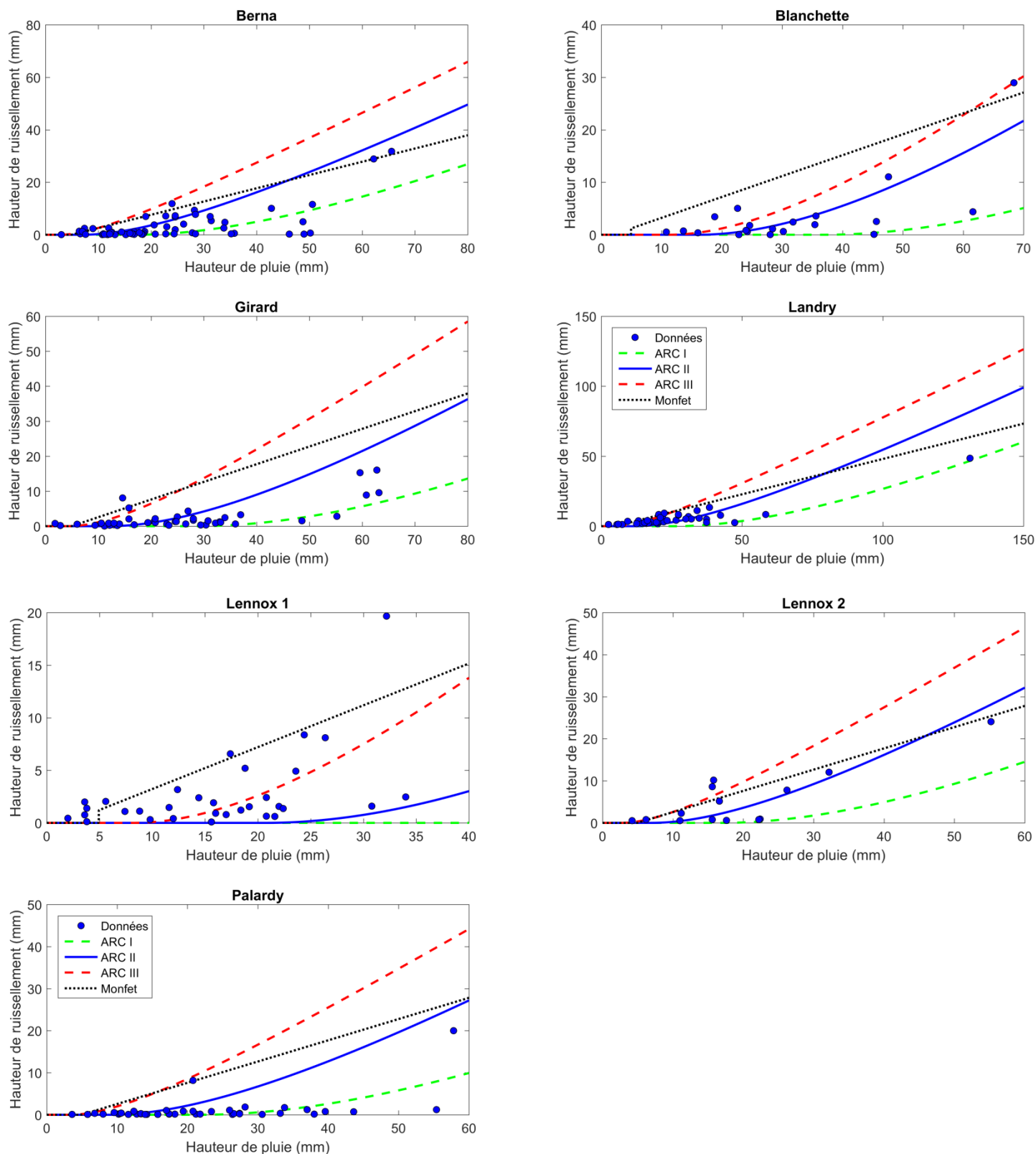
Figure 5.3 – Hauteur de ruissellement (mm) en fonction de la hauteur de pluie (mm) aux sites sous étude. Les courbes correspondent à la Méthode SCS originelle (ARC I, II et III) et les points aux valeurs mesurées aux différents sites. Les régressions de Monfet sont également présentées.
