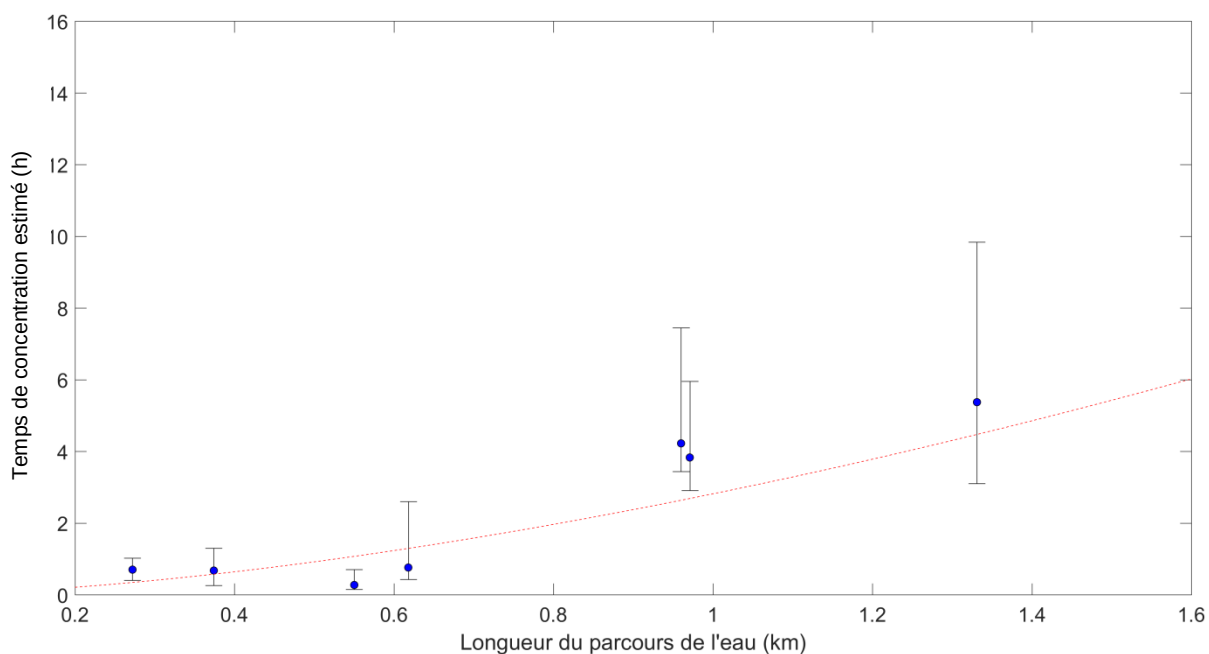
Figure 4.10 - Temps de concentrations estimés à partir des observations (médianes des valeurs obtenues par la méthode T_p en chaque site) et par la régression basée sur la formulation de Sheridan modifiée ( T_C = 2.8 L^{1.6} ; traits pointillés). Les traits verticaux délimitent les 25 e et 75 e percentiles des valeurs des temps de concentration estimées par la méthode T_p en chacun des sites.
