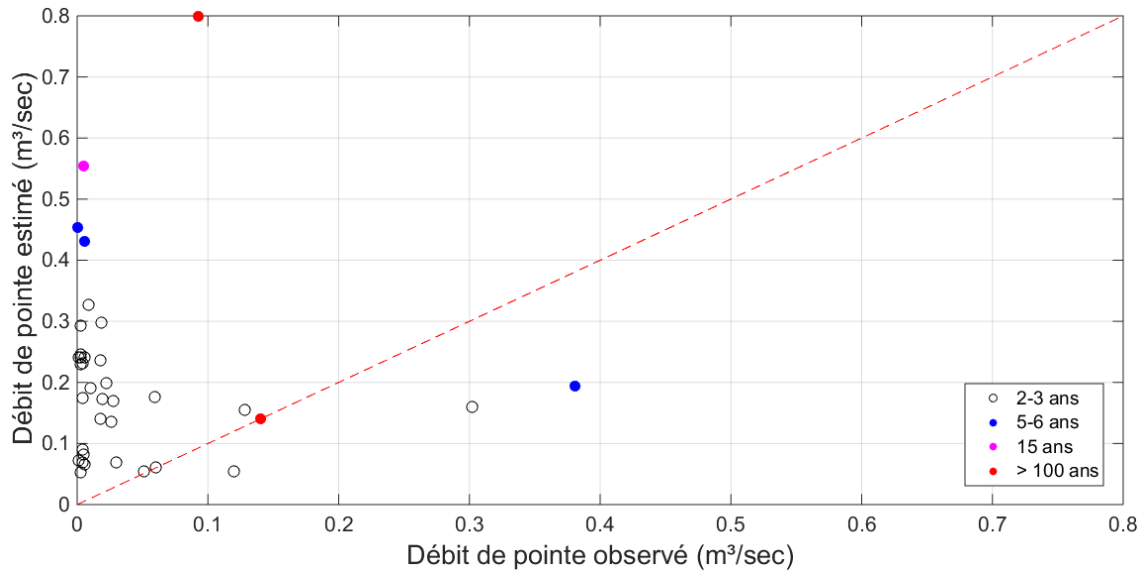
Figure 6.3 – Comparaison des débits de pointe observés et des débits de pointe estimés à partir de la méthode rationnelle en considérant le temps de concentration médian de la méthode d'estimation des temps de concentration T_p . La période de retour de chacun des événements de pluie est également indiquée. La ligne pointillée rouge représente la droite de pente 1.
