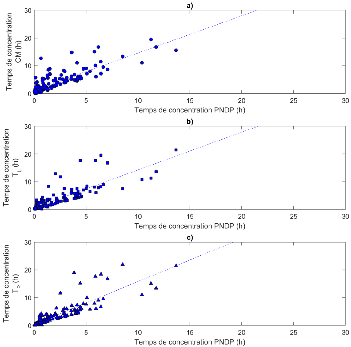
Figure 4.7 - Régressions des valeurs estimées à partir des méthodes : a) CM; b) T_L ; c) T_P en fonction des valeurs estimées à partir de la méthode PNDP. Les courbes en pointillés correspondent aux régressions linéaires correspondantes (voir Tableau 4.9 pour les valeurs des paramètres de régression).
