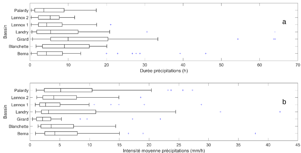
Figure 4.2 - Box plots des : a) durées, b) des intensités moyennes de tous les événements de pluie/débit (248 événements au total).
