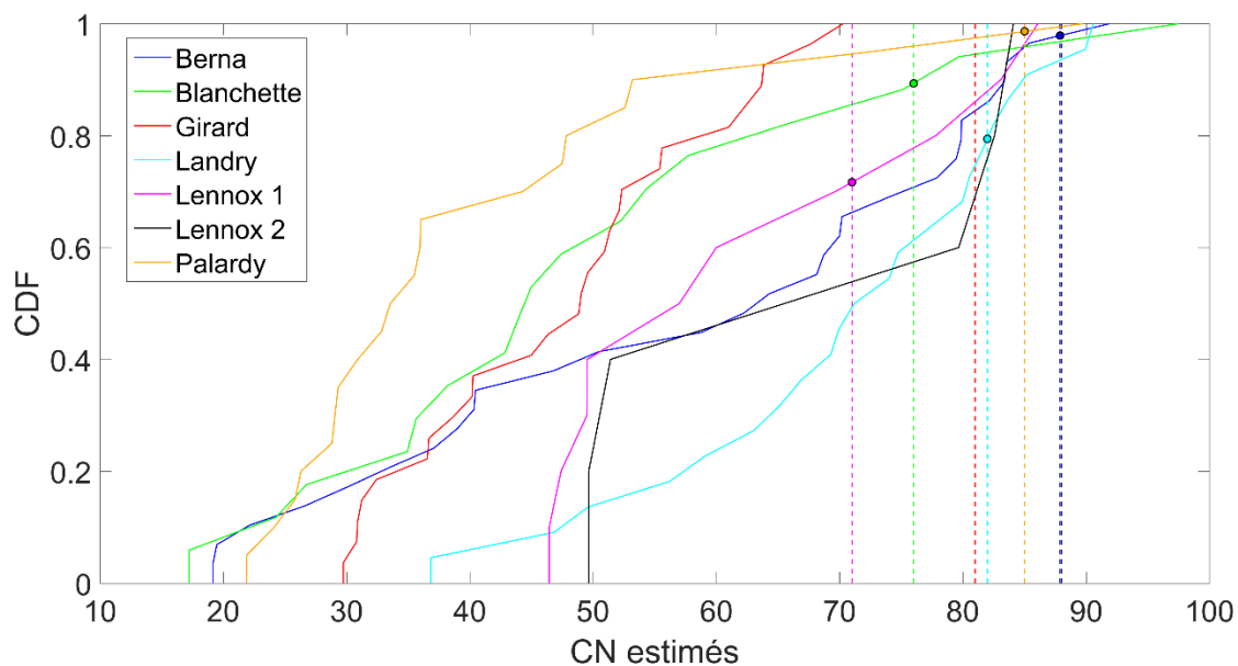
Figure 5.5 – Cumulative Distribution Function (CDF) des valeurs de CN des différents événements aux différents sites. Les lignes verticales correspondent aux valeurs de CN de la Méthode SCS originelle (ARC II) et les points sont à l'intersection entre ces valeurs et les CDF du site correspondant. La valeur de \lambda = 0.03 a été considérée.
