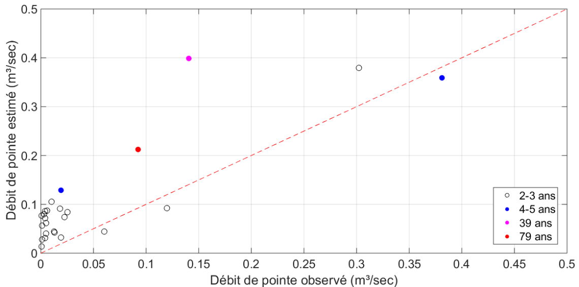
Figure 6.6 – Comparaison des débits de pointe observés et des débits de pointe estimés à partir de la MHT modifiée, considérant le temps de concentration obtenu avec l'équation de Sheridan modifiée, selon la période de retour de chacun des événements pluie/débit (la ligne en rouge représente la droite de pente 1).
