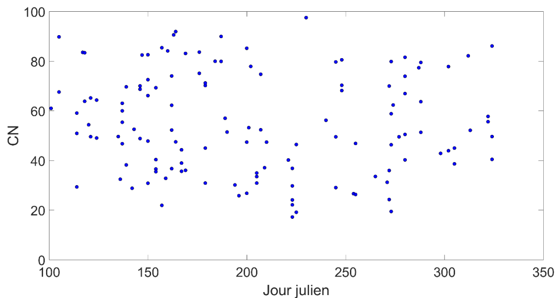
Figure 5.9 – Valeurs de CN estimées à partir de la méthode SCS ajustée en fonction du jour julien où est survenu l'événement de pluie/débit.
